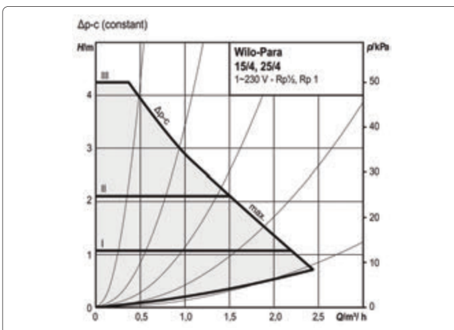
Kennlinien Wilo-Para, konstanter Differenzdruck
