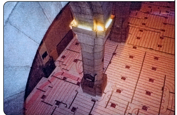
MB-Systemverlegung von oben
